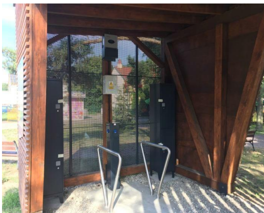
Fotografia 28-29. Wiata serwisowa w Poddąbiu (widoczny punkt ładowania rowerów elektrycznych i szafki bagażowe).
