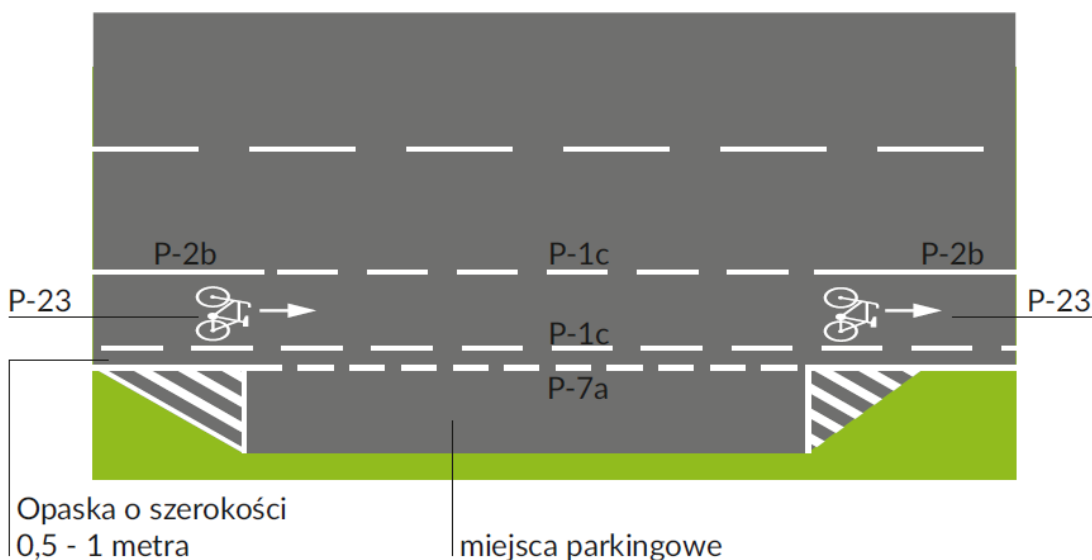
Rysunek 29. Przykład prowadzenia pasa rowerowego wzdłuż wyznaczonego pasa do parkowania pojazdów / miejsc do parkowania. Źródło: opracowanie własne.
