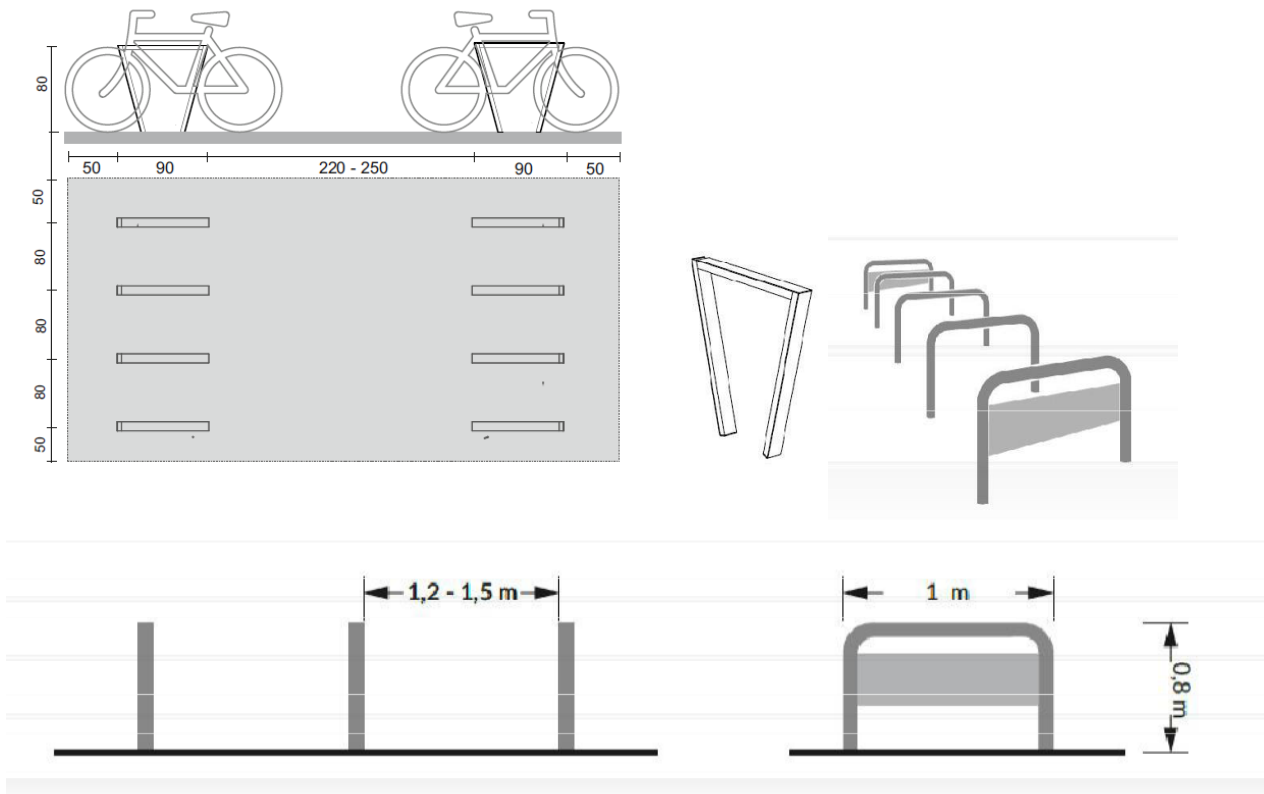
Rysunek 74. Rekomendowany wygląd i rozmieszczenie stojaków rowerowych na miejscach odpoczynku. Źródło: Opracowanie własne, materiały Urzędu Marszałkowskiego Województwa Pomorskiego.
