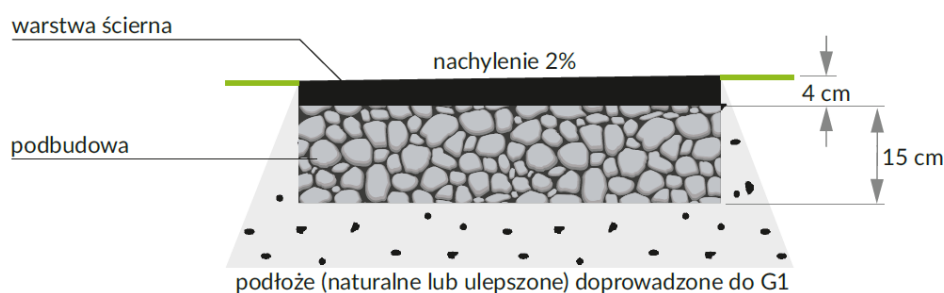
Rysunek 37. Konstrukcja drogi rowerowej o nawierzchni bitumicznej (jedna warstwa asfaltu).
