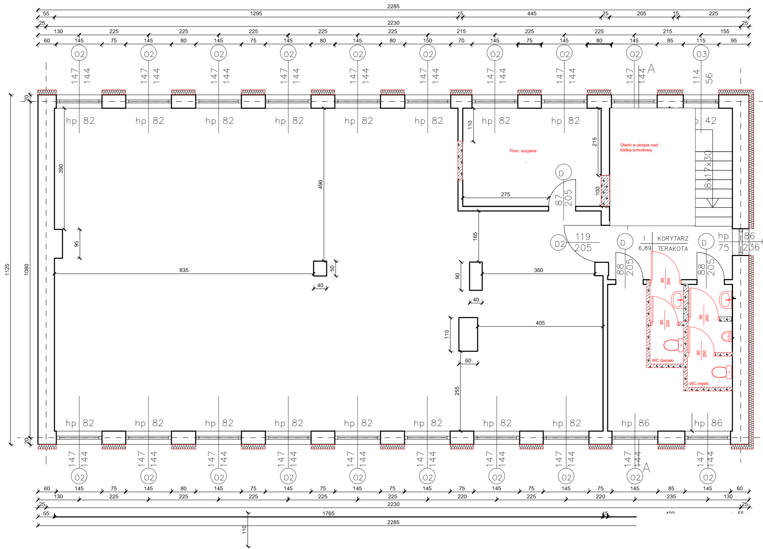
RZUT PIĘTRA
