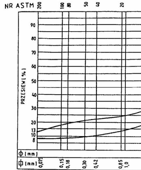
Rys. 5. Krzywe graniczne uziarnienia mieszank mineralnych SMA od 0 mm do 12,8 mm
