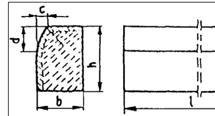
Rys. 1. Wymiarowanie krawężników i oporników
