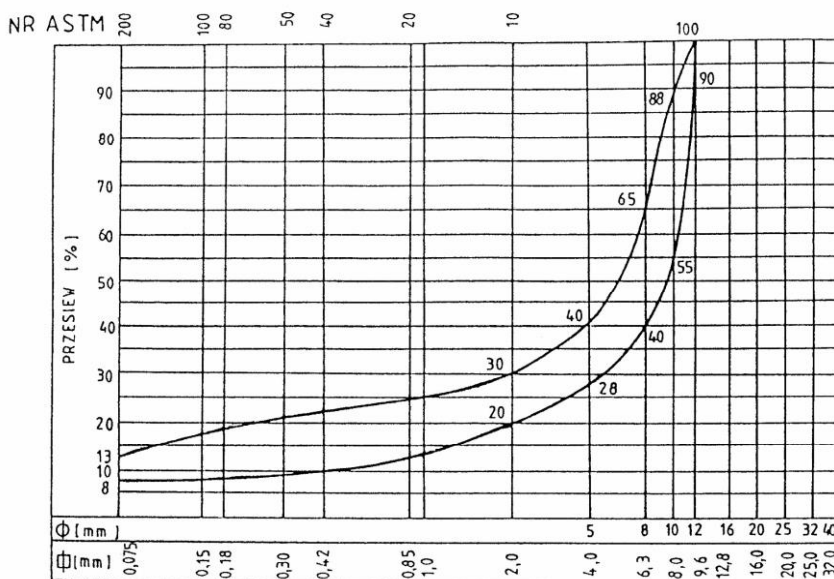
Rys. 4. Krzywe graniczne uziarnienia mieszank mineralnych SMA od 0 mm do 9,6 mm
