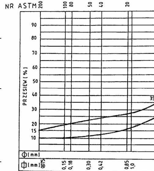
Rys. 1. Krzywe graniczne uziarnienia mieszank mineralnych SMA od 0 mm do 4 mm
