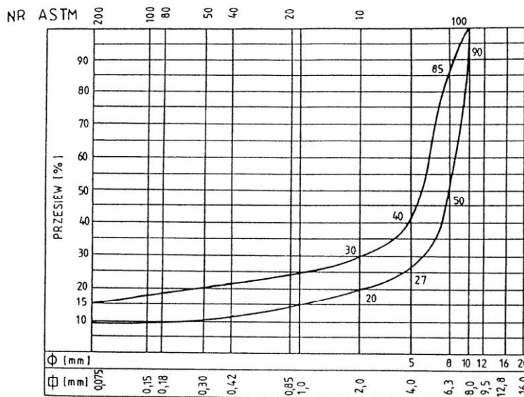
Rys. 3. Krzywe graniczne uziarnienia mieszank mineralnych SMA od 0 mm do 8 mm
