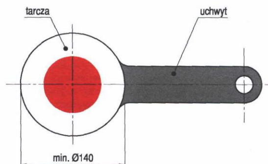
Rys. 14.2.1. Tarcza do zatrzymywania pojazdów
