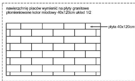
Detal P3 - nawierzchnia - 1:100
