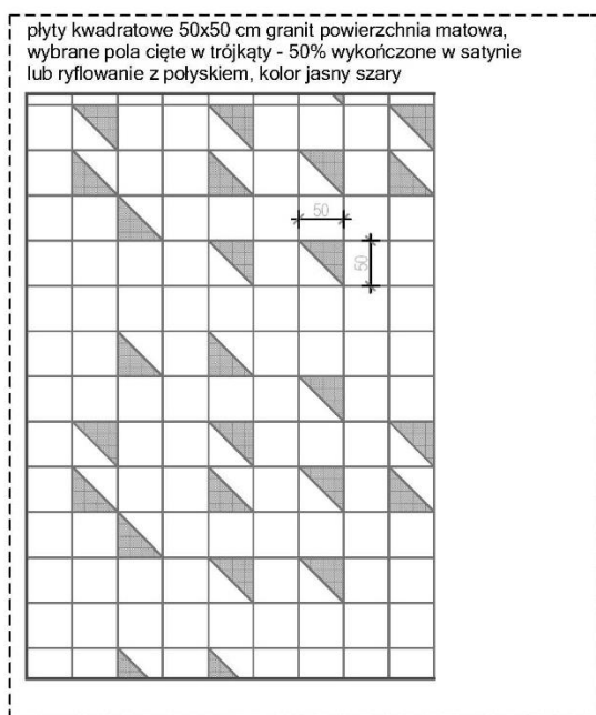
Detal P1 - nawierzchnia - 1:100
