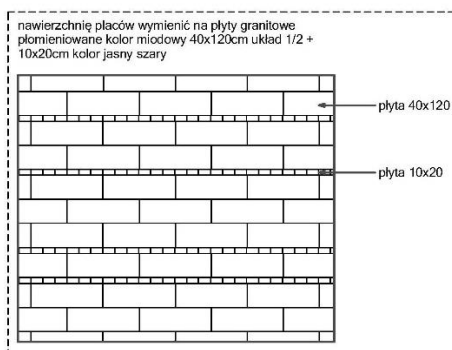
Detal P6 - nawierzchnia - 1:100
