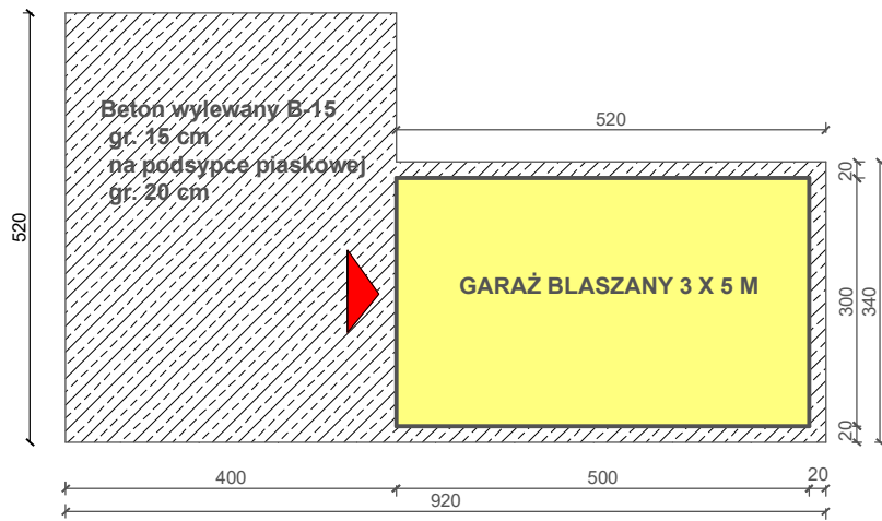
RZUT PRZYZIEMIA skala 1 : 100
