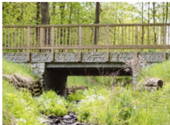
Gęsto szczelbowana barierka na moście. Źródło: Archiwum CKPŚ.
