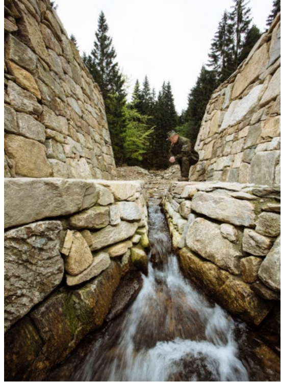
V-kształtny przelew wody ze zbiornika przeciwpowodziowego umożliwiający przejście rumowiska i samoczynne napełnianie i opróżnianie obiektu - Nadleśnictwo Międzylesie. Źródło: Archiwum CKPŚ. (rys. z prawej strony)
