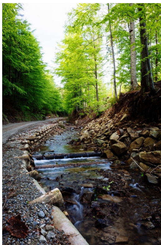
Poniżej progu widoczne są dwa „baseny”, prog pośrodku i gurt. Niestety próg nie ma przelewu na małą wodę. Źródło: Archiwum CKPŚ.
