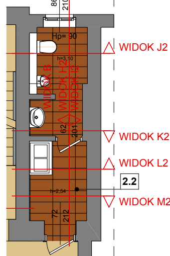
WIDOK K2
