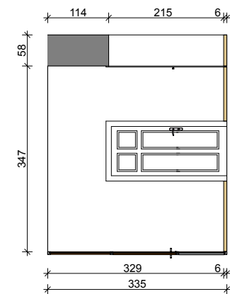
WIDOK F2
