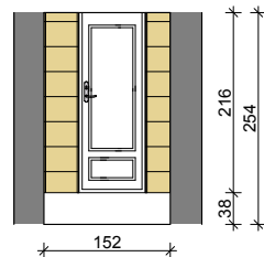
WIDOK M2
