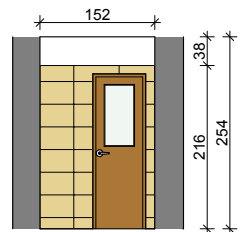
WIDOK L2
