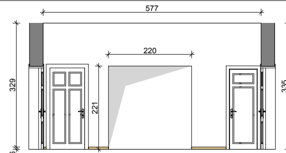
WIDOK E2
