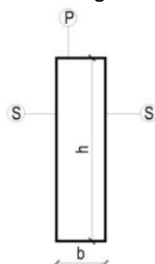
Rysunek A. Kształt kamiennego obrzeża chodnikowego
