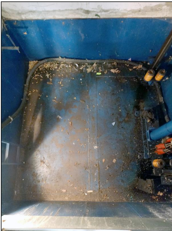
Podszycie z wanną stalową
