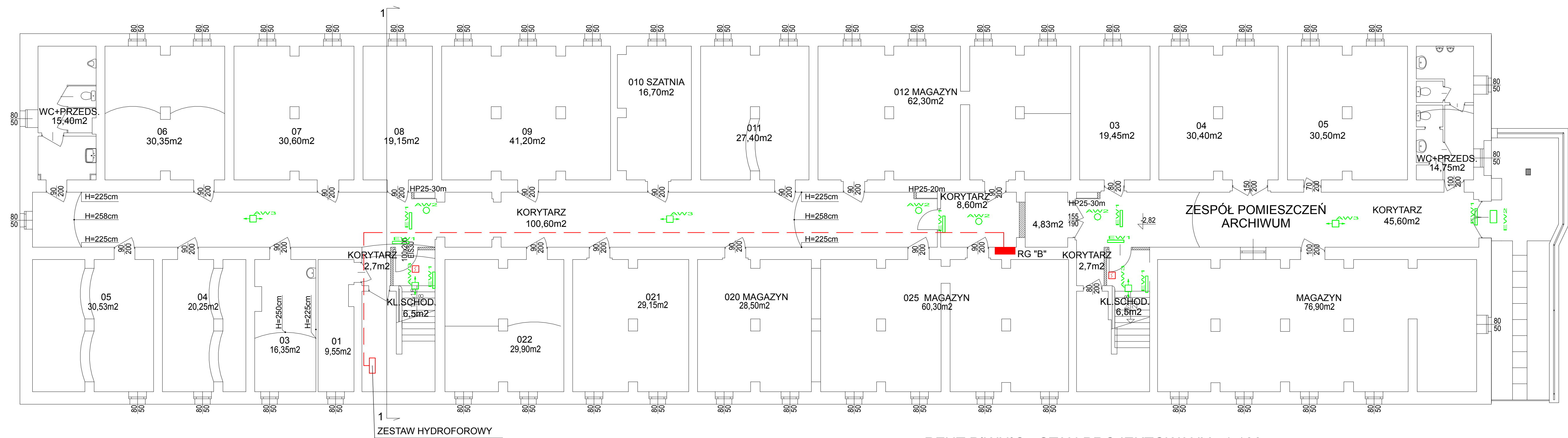
RZUT PIWNIC - STAN PROJEKTOWANY 1:100 BUDYNEK "B"
