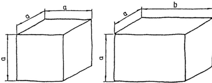
Rysunek 1. Kształt kostki regularnej normalnej i łącznikowej
