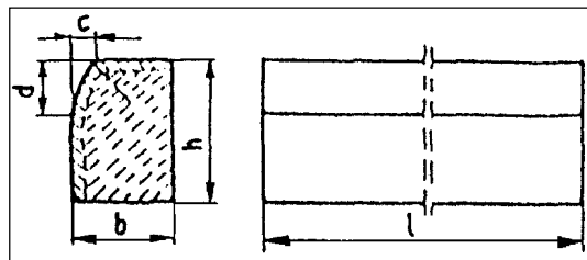
Rys. 1. Wymiarowanie krawężników i oporników
