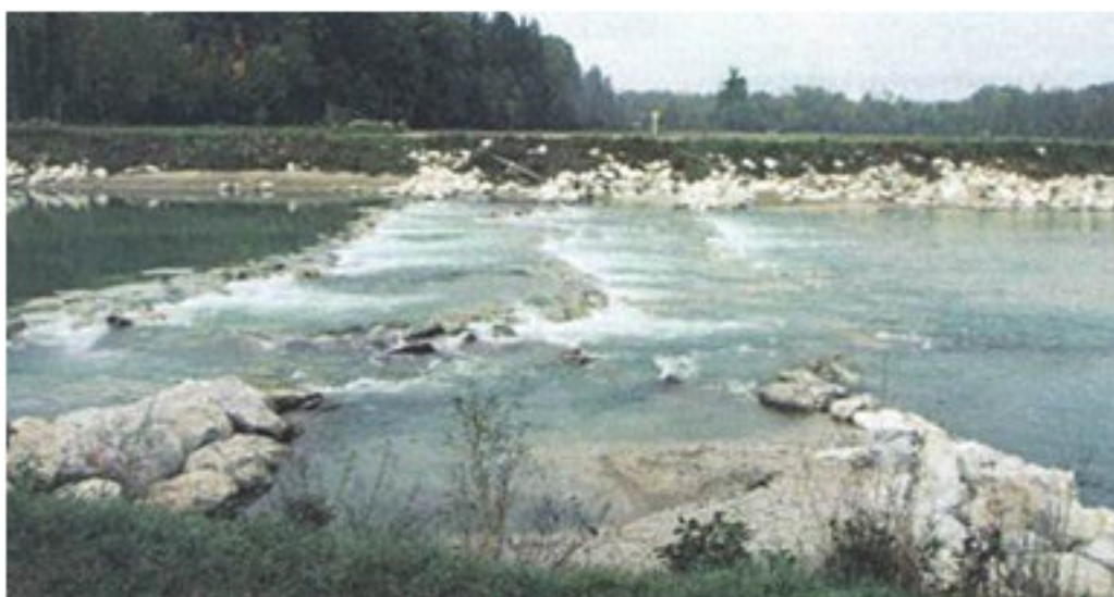
Fot. 7. Bystrze kaskadowe na rzece podgórskiej (Jelonek 2008)
