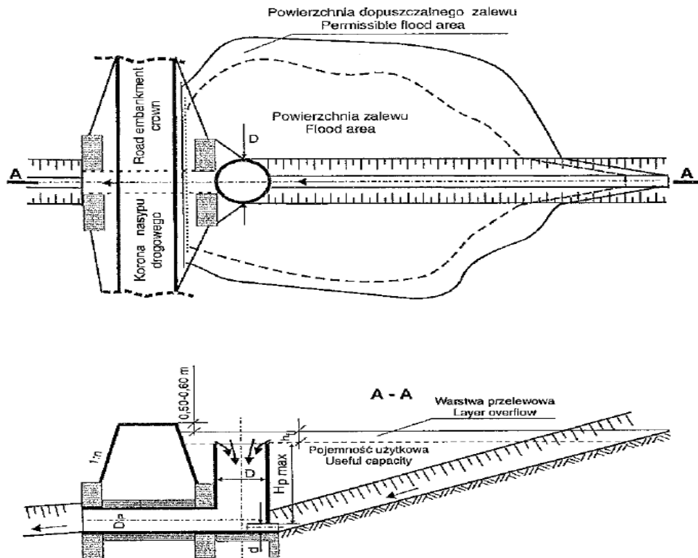
Opóźniacz odpływu, rzut z góry przekrój podłużny (J. Paluch 2005)
