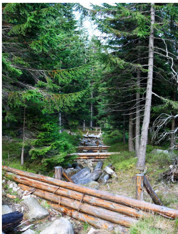
Dawny, zrenaturyzowany szlak zrywkowy zabezpieczony przed spływem powierzchniowym.
