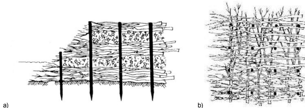
Brzegosłon krzyżowy a - przekrój poprzeczny, b – rzut z góry (Begemann i Schiechtel 1999)
