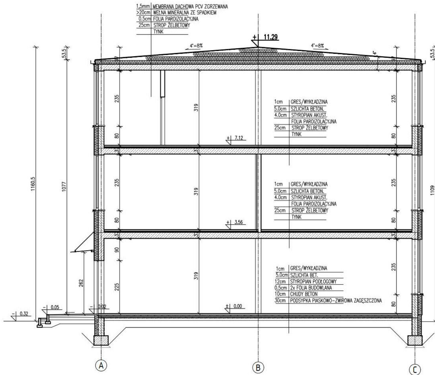
PRZEKRÓJ A-A
