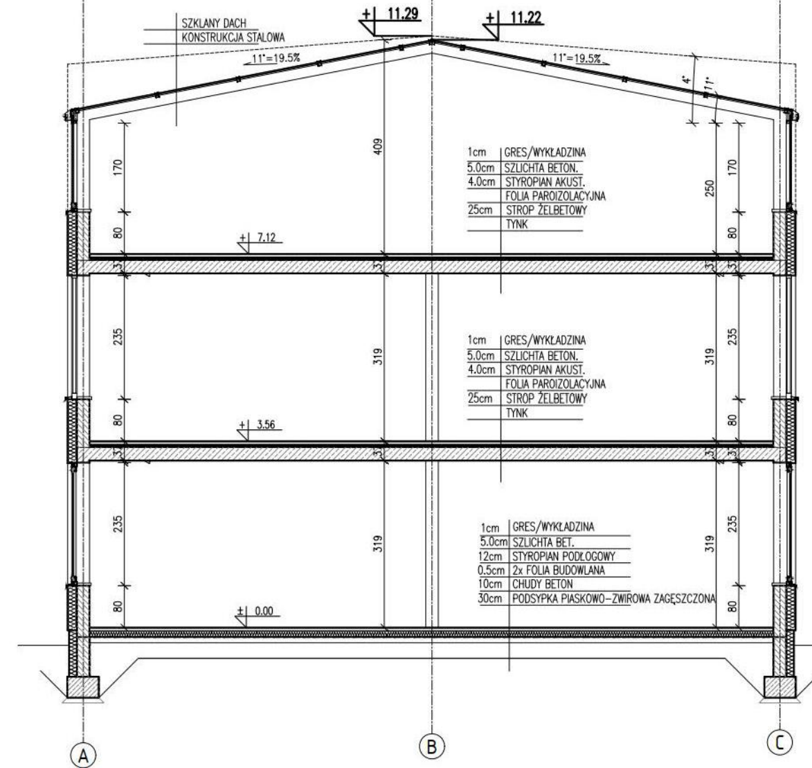
PRZEKRÓJ C-C
