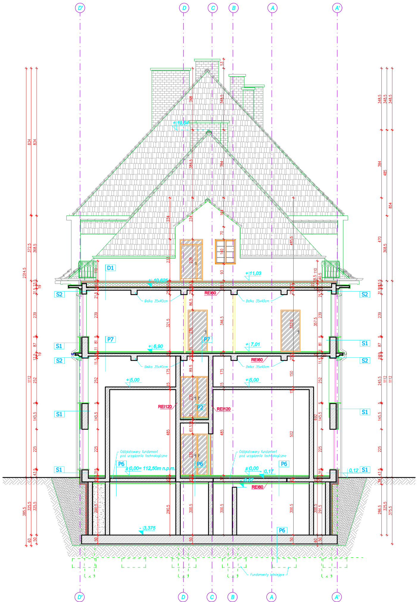
PRZEKRÓJ F-F
