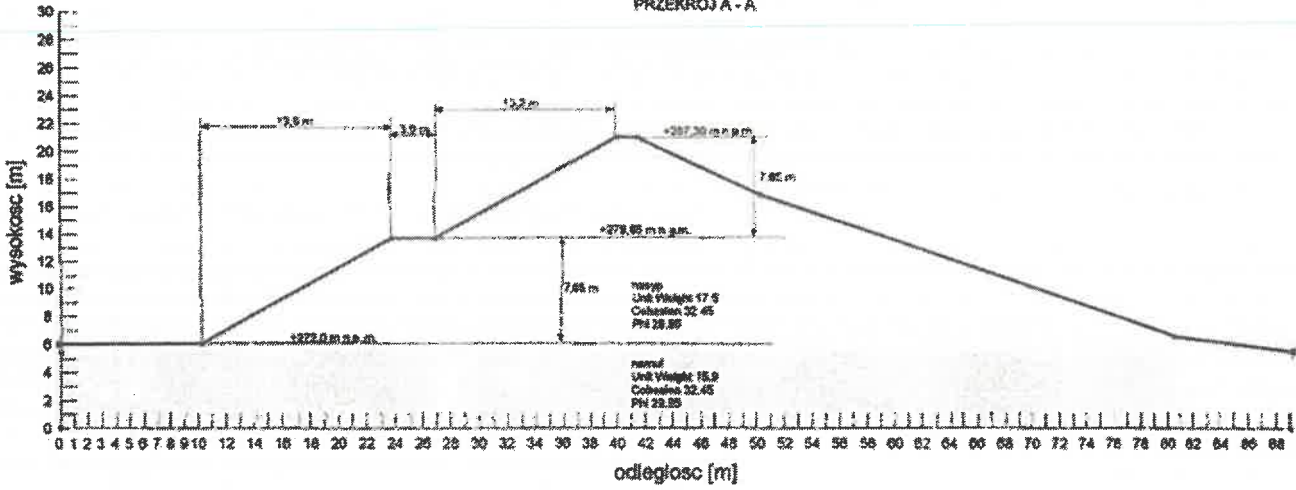
PRZEKROJ A - A
