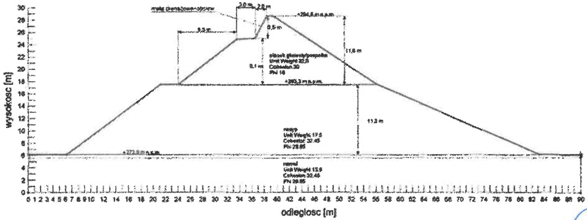
PRZEKROJ B - B'
