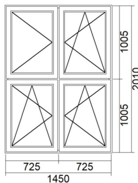
Rysunek nr 1. Orientacyjne wymiary okna oraz wymagane przez zamawiającego funkcjonalności (sposób otwierania).
