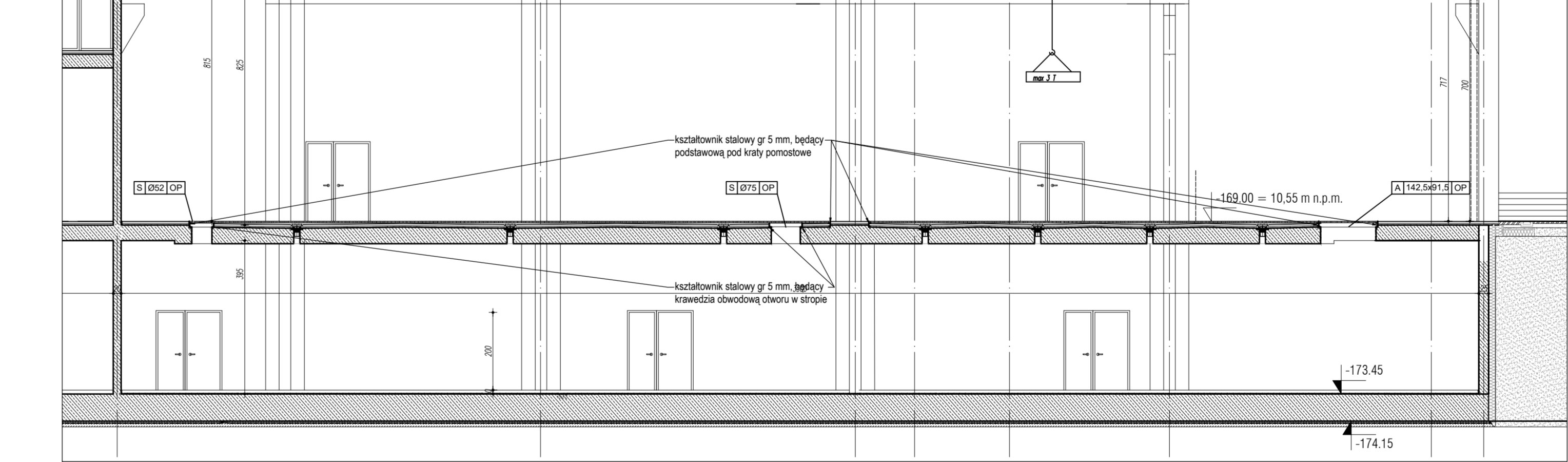
PRZEKRÓJ PRZEZ STROP POM. P9/PODŁOGĘ POM. 0.17 - WPUSY I OTWORY W STROPIE SKALA 1:100
