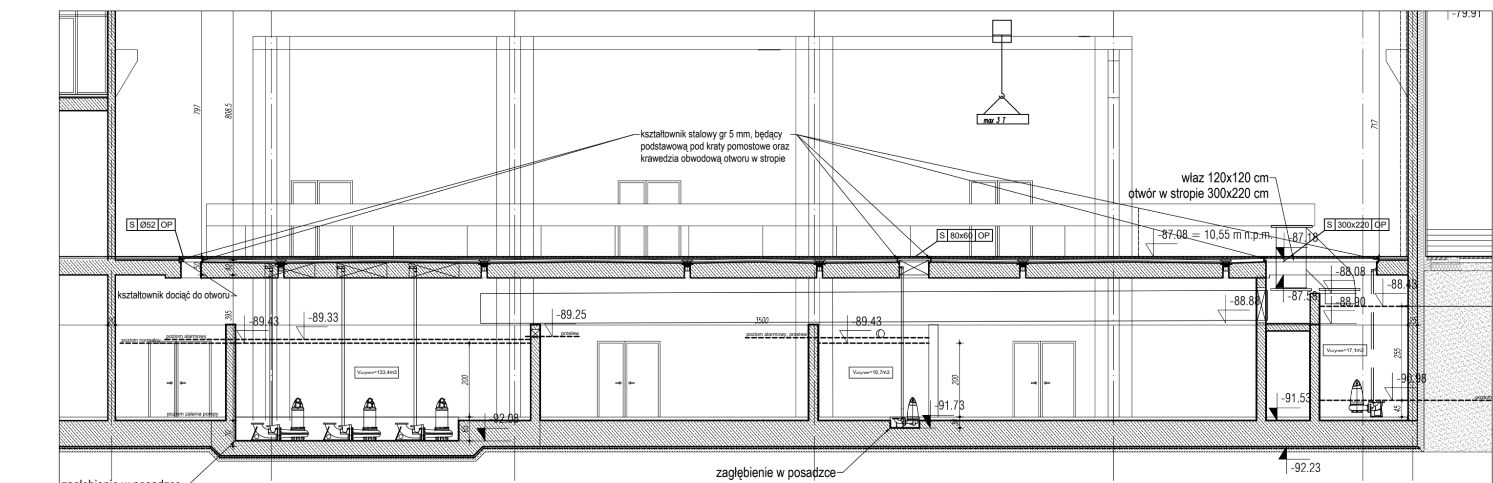
PRZEKRÓJ PRZEZ ZBIORNIKI WODY POM. P9 ORAZ STROP POM. P9/PODŁOGĘ POM. 0.17 SKALA 1:100
