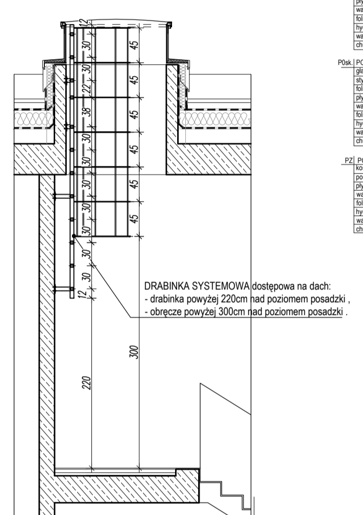
DETAIL DRABINY WYŁAZOWEJ SKALA 1:50
