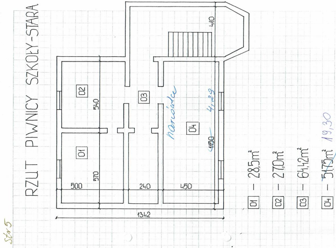
rys. 1 - schemat piwnic
