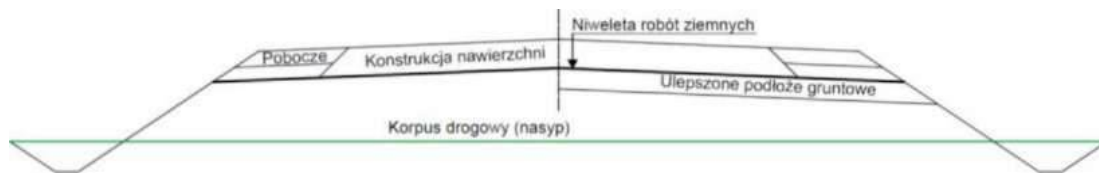
Rysunek 1.1. Lokalizacja niwelety robót ziemnych
