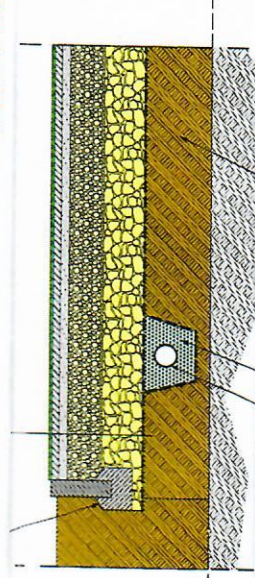
PRZEKRÓJ NAWIERZCHNI Z TRAWY SYNTETYCZNEJ BOISKA WRAZ Z DRAŻĄŻEM
