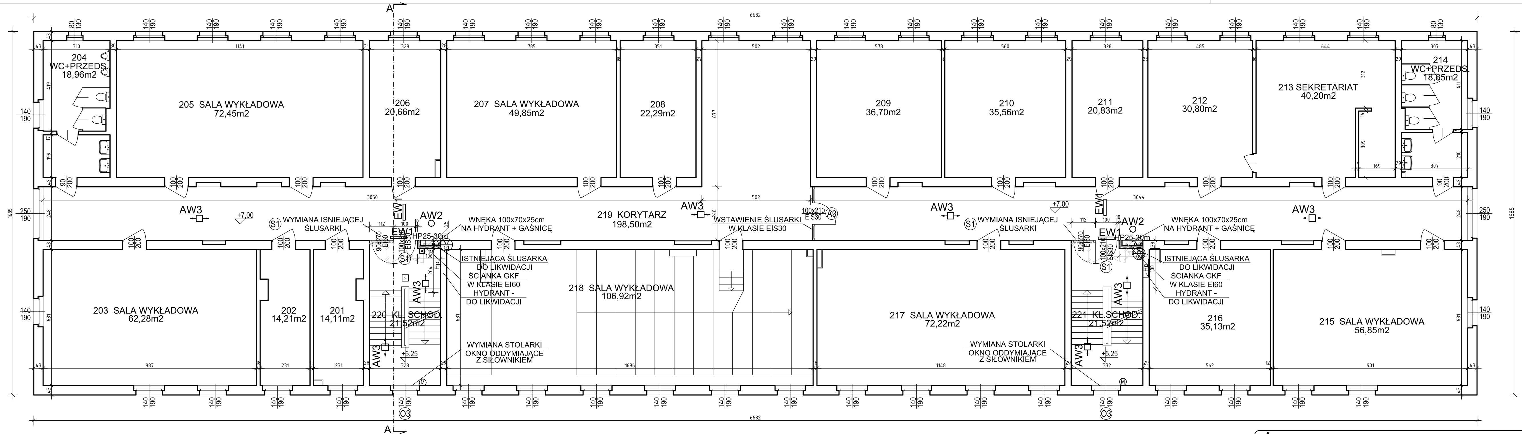
RZUT II PIĘTRA - STAN PROJEKTOWANY 1:100 BUDYNEK "B"
