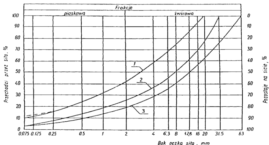
Rysunek 1. Pole dobrego uziarnienia kruszyw przeznaczonych na podbudowy wykonywane metodą
