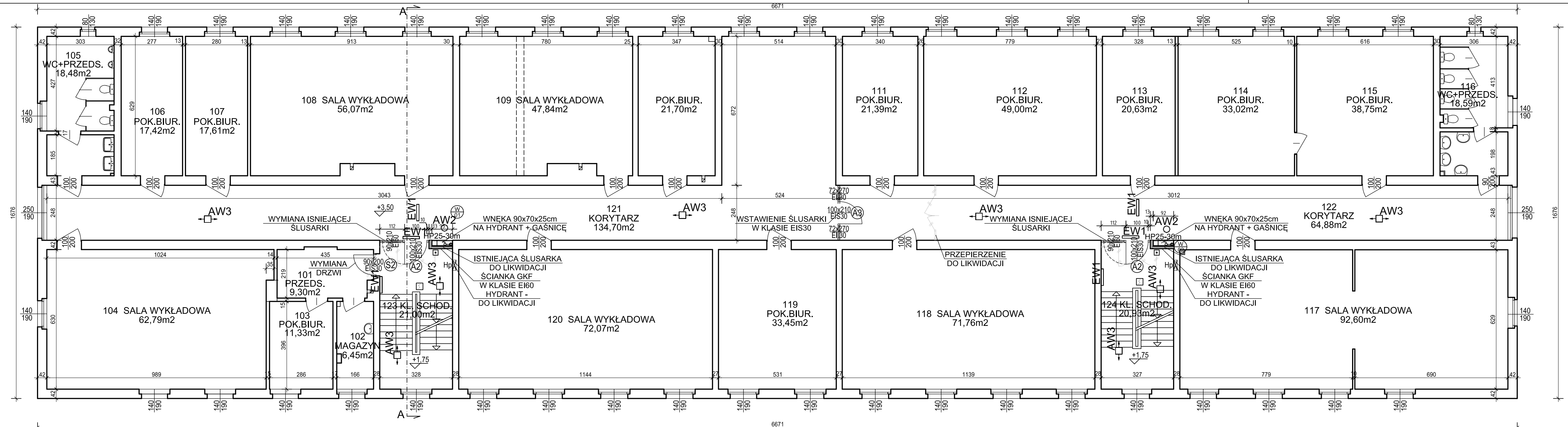
RZUT I PIĘTRA - STAN PROJEKTOWANY 1:100 BUDYNEK "D"
