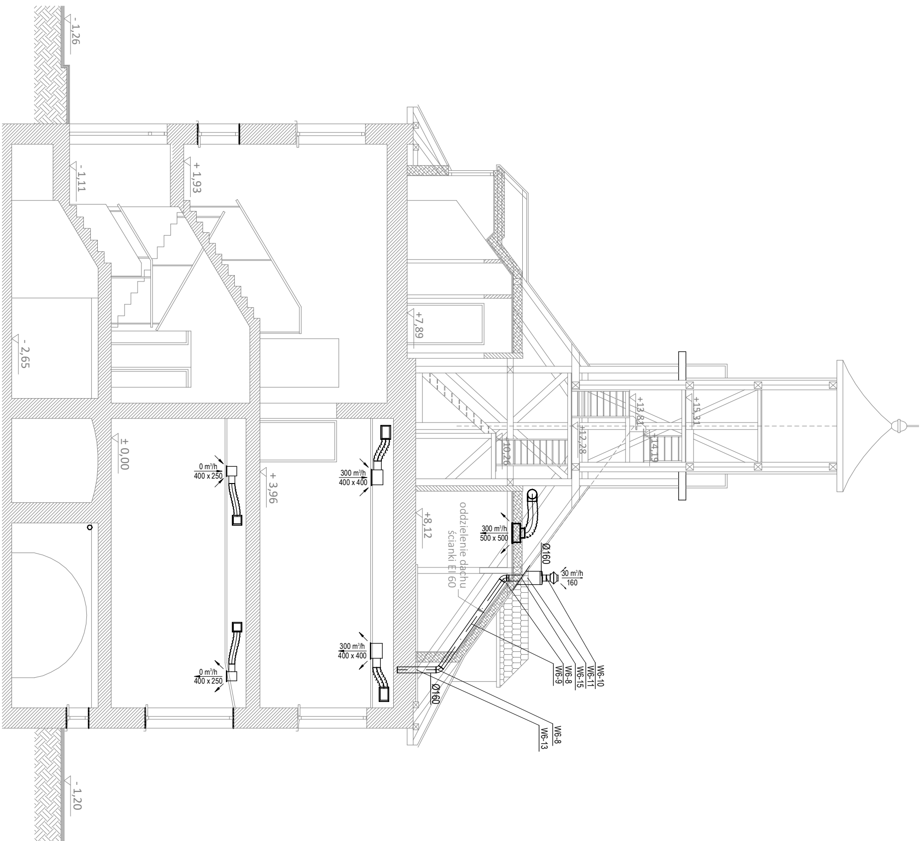
PRZEKRÓJ A-A skala 1:100
