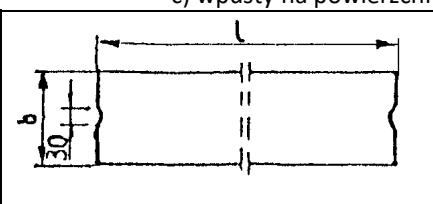
Rys. 1. Wymiarowanie krawężników
