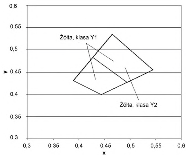
Rys.2. Współrzędne chromatyczości x,y dla barwy żółtej oznakowania
