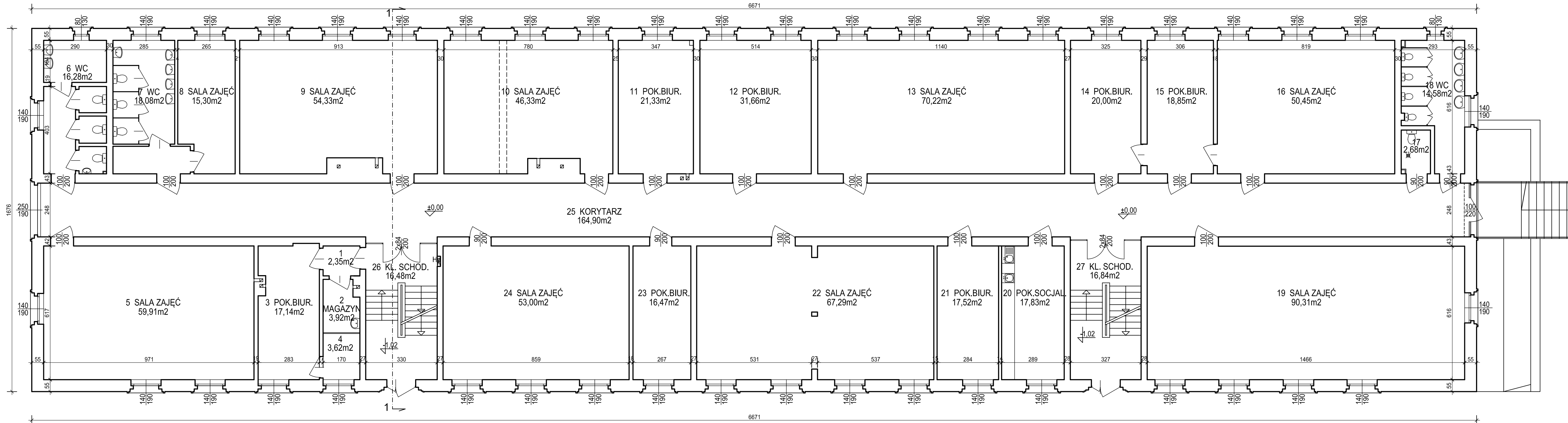
RZUT PARTERU - STAN ISTNIEJĄCY 1:100 BUDYNEK "D"
