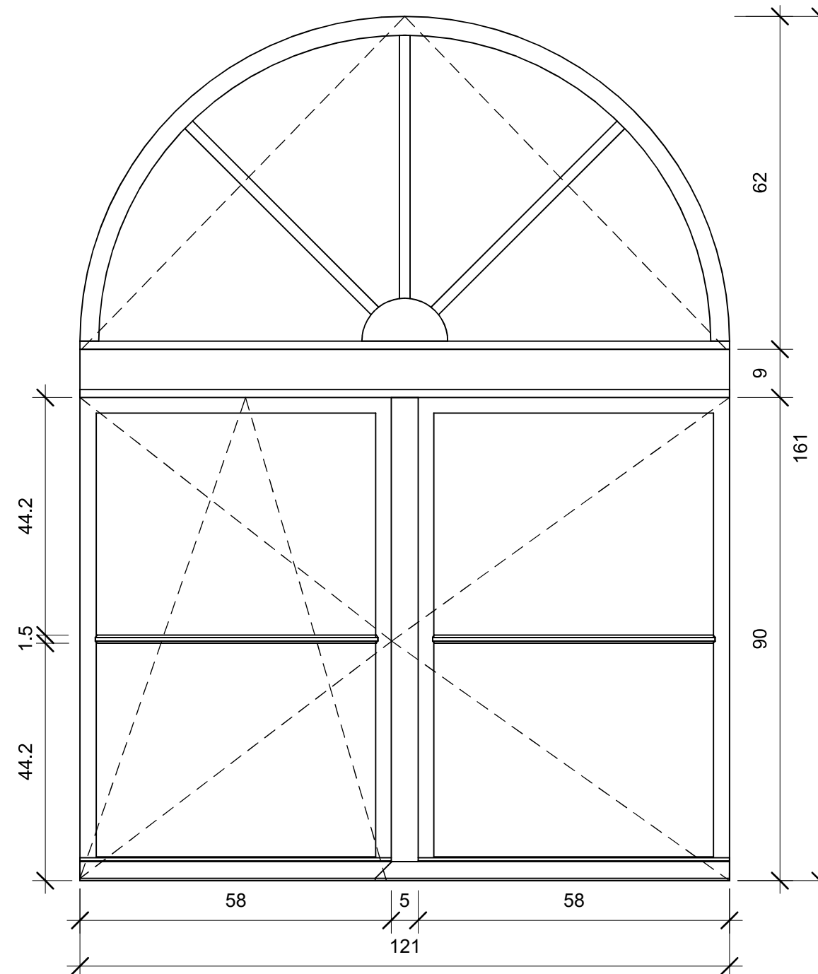
SCHEMAT PODZIAŁU OKNA I PROJEKT OTWIERANIA
