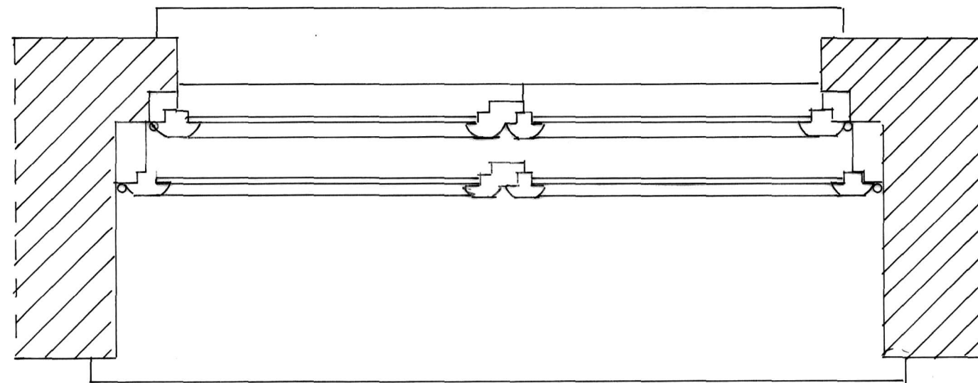
ISTNIEJĄCY PRZEKRÓJ OKNA SKRZYNKOWEGO
