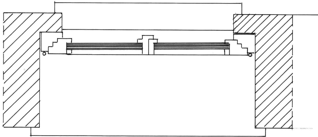
PROJEKTOWANY PRZEKRÓJ OKNA 3-SZYBOWEGO
