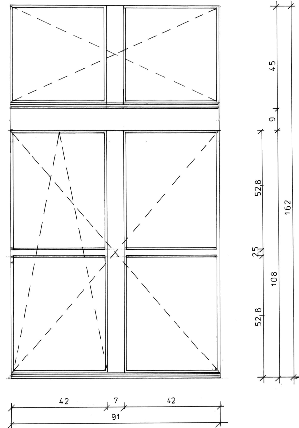
SCHEMAT PODZIAŁU OKNA I PROJEKT OTWIERANIA
