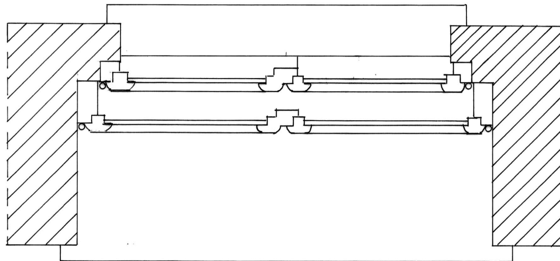
ISTNIEJĄCY PRZEKRÓJ OKNA SKRZYNKOWEGO
