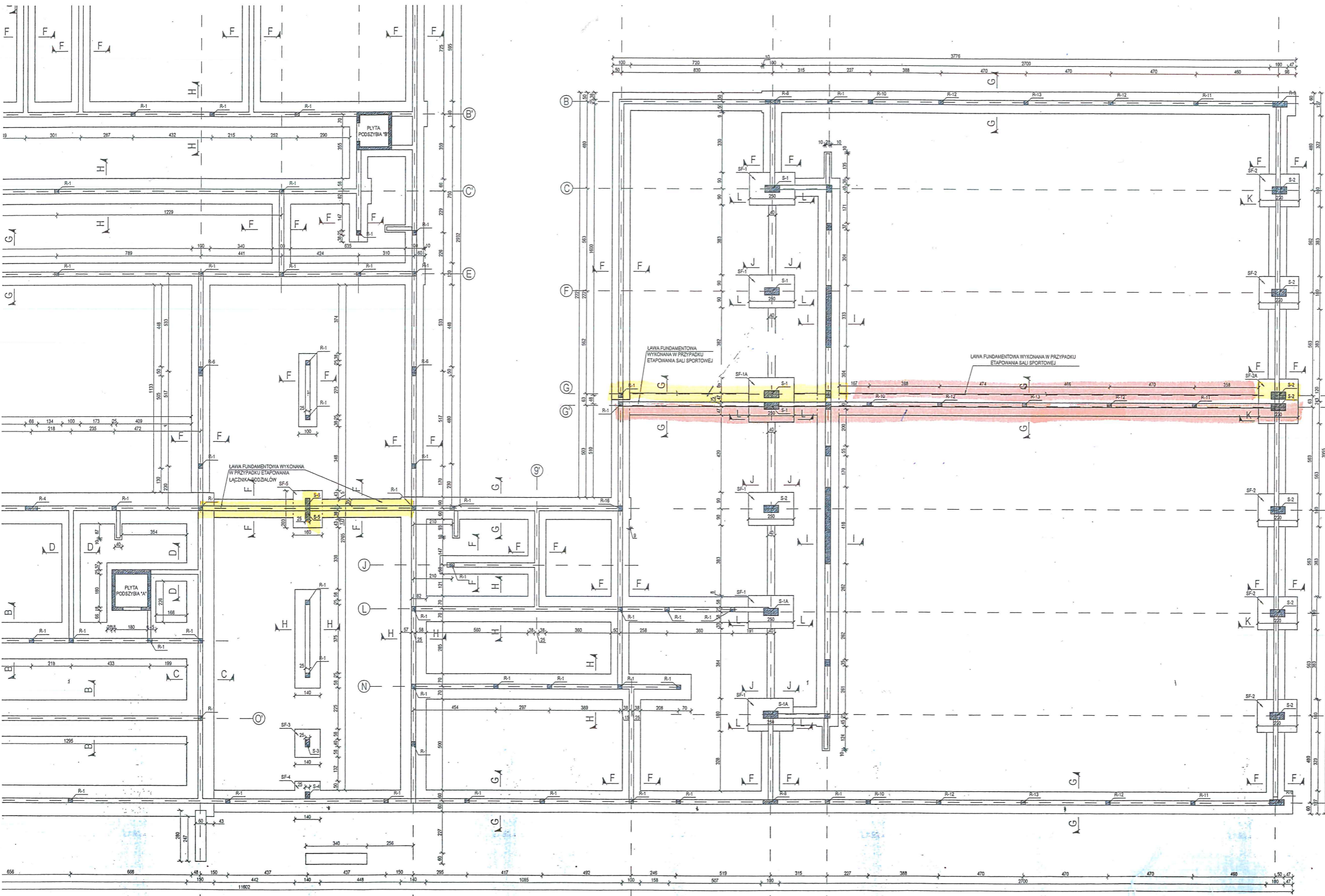
RYSUNEK POGLĄDOWY NR 2 Planowani do wykonania zakres robót fundamentowych (elementy opisane w projekcie budowlanym jako: do wykonania (bądź odstąpienie od wykonania) w razie etapowania zadania) - fundamenty przewidziany do wykonania - fundamenty od wykonania którego odpuszczamy
