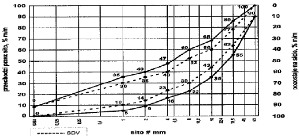
Rys. 12. Mieszanka niezwiązana 0/45 do warstwy podbudowy zasadniczej
