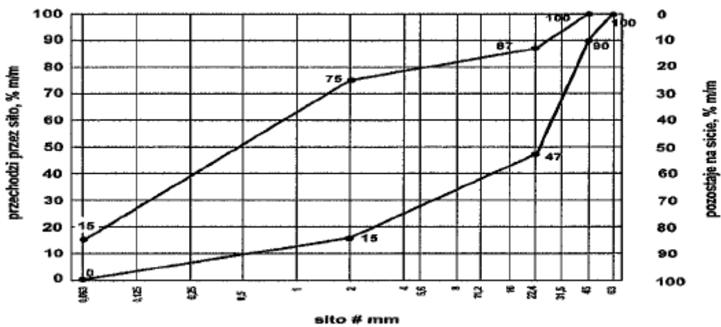
Rys. 6. Mieszanka kruszyw 0/45 do górnej warstwy podłoża ulepszonego
