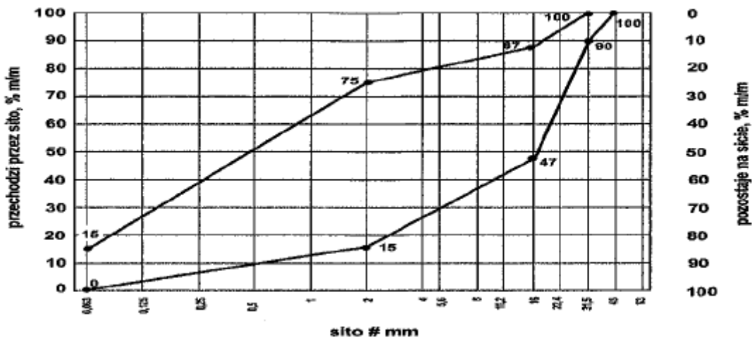
Rys. 5. Mieszanka kruszyw 0/31,5 do górnej warstwy podłoża ulepszonego
