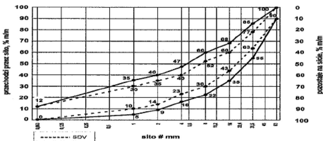
Rys. 10. Mieszanka niezwiązana 0/63 do warstwy podbudowy-pomocniczej Oprócz wymagań podanych na rysunkach od 8 do 10, wymaga się, aby 90 % uziarnień mieszanek zbadanych w ramach ZKP w okresie 6 miesięcy spełniało wymagania kategorii podanych w tablicach 2 i 3, aby zapewnić jednorodność i ciągłość uziarnienia mieszanek.
