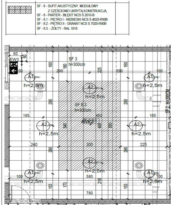
rys. nr 601 „rzut sufitów parter – przedszkole”
