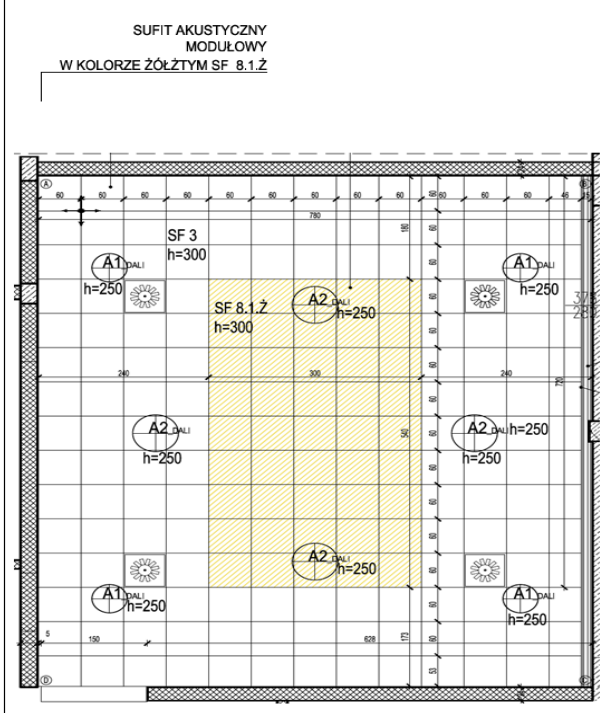
rys. nr 720 „Przedszkole sala zajęć P. 031”
