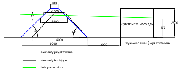
Obwałowanie Placu składowego TAJWAN - Przekrój 4
