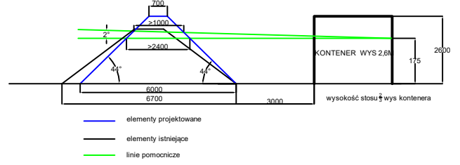
Obwałowanie Placu składowego TAJWAN - Przekrój 3
