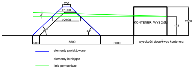
Obwałowanie Placu składowego TAJWAN - Przekrój 1
