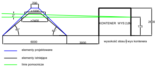
Obwałowanie Placu składowego TAJWAN - Przekrój 2
