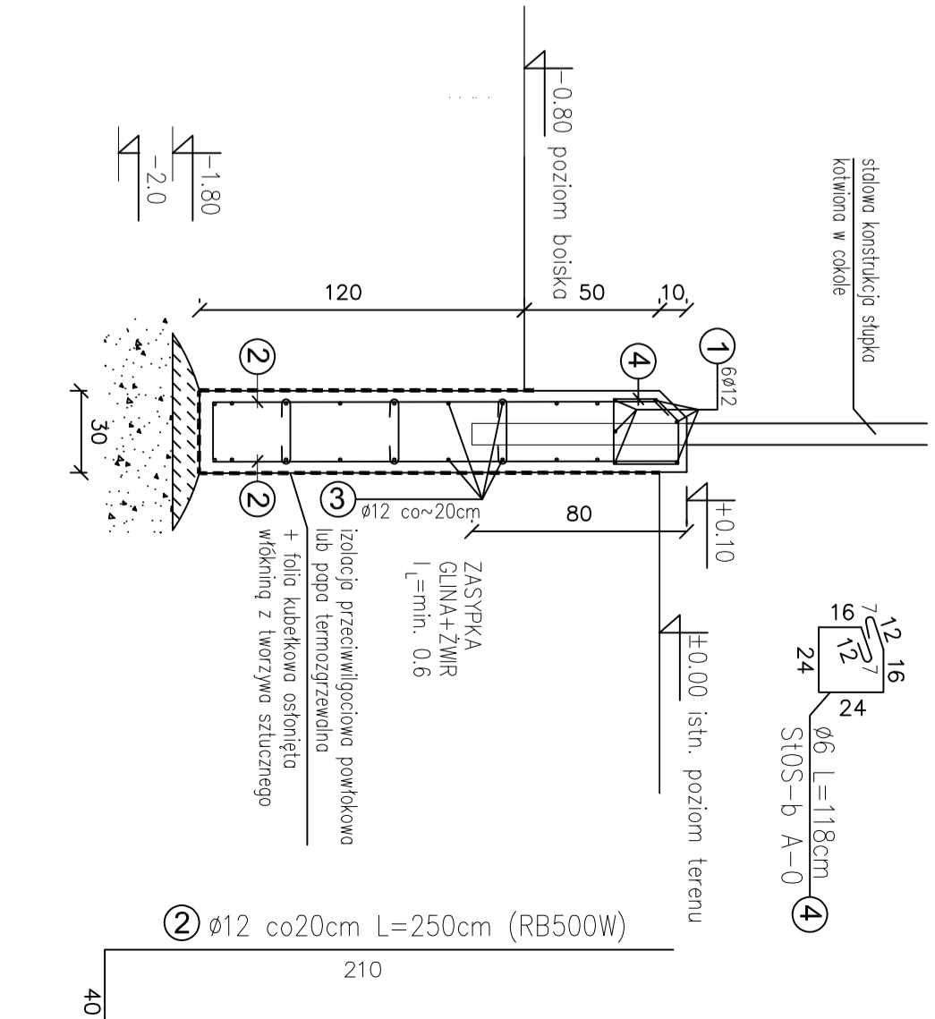
DETAL COKOKU 1:25
