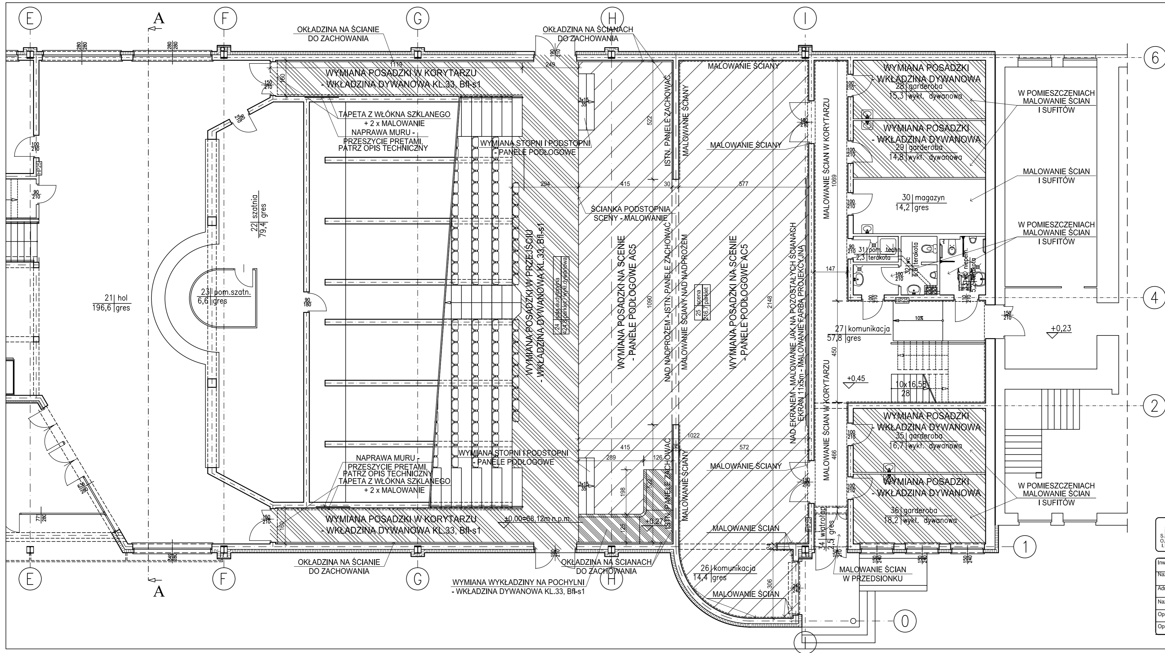
Państwowa Uczelnia Stanisława Staszica budynek Auditorium Maximum "F" RZUT PARTERU - stan projektowany Skala 1:100
