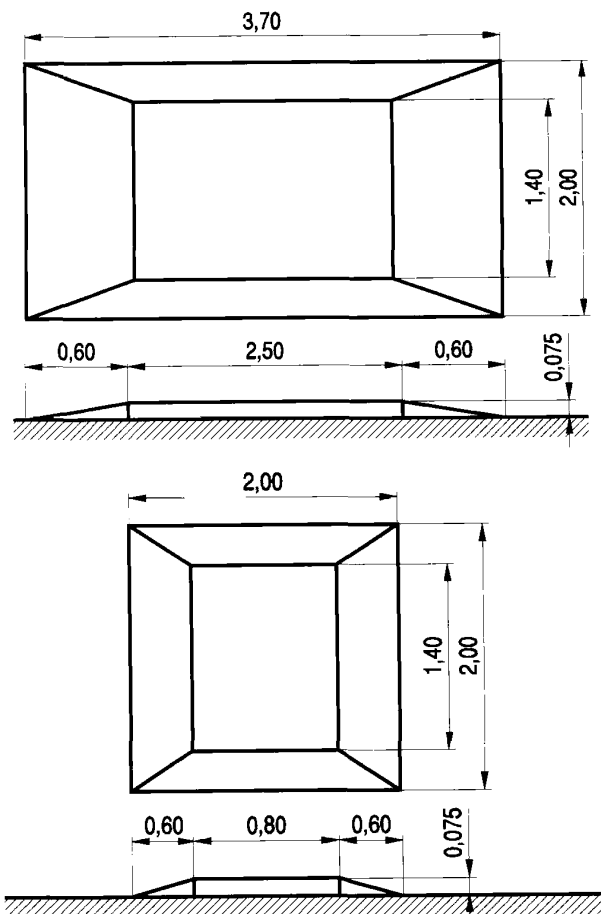
Rys. 2. Przykłady wymiarowania progów zwalniających wyspowych (wg [23])
