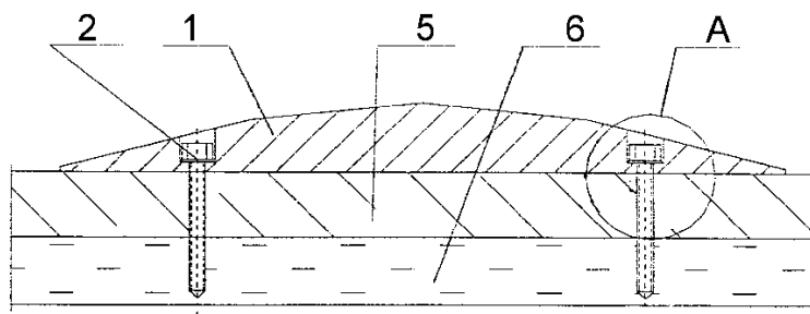
Rys. 4. Przykład umocnienia progów do nawierzchni jezdni
