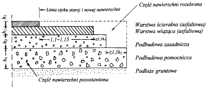
Rys. 2. Konstrukcja połączenia starej i nowej nawierzchni
