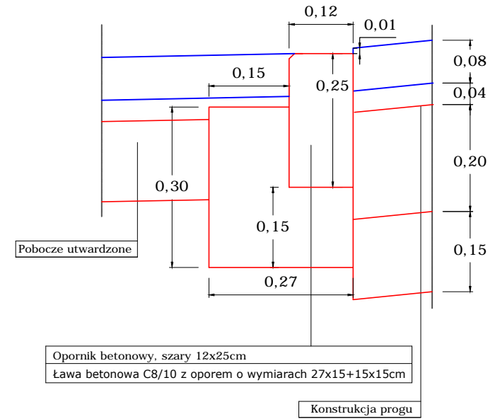
Szczegół konstrukcyjny B- opornik betonowy (pomiędzy poboczem a progiem)
