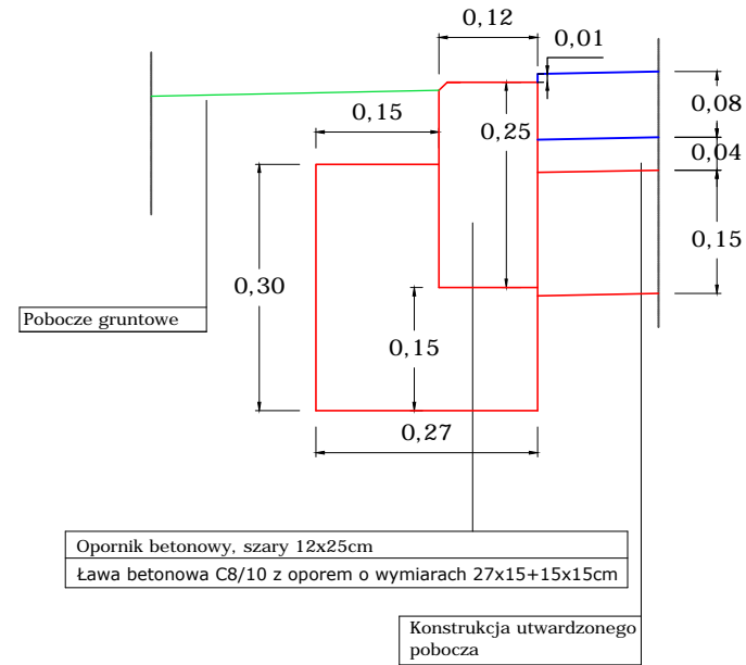
Szczegół konstrukcyjny A- opornik betonowy (krawędź utwardzonego pobocza)
