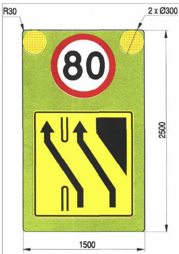
Rys. 21. Tablica wczesnie ostrzegajaca U-27
