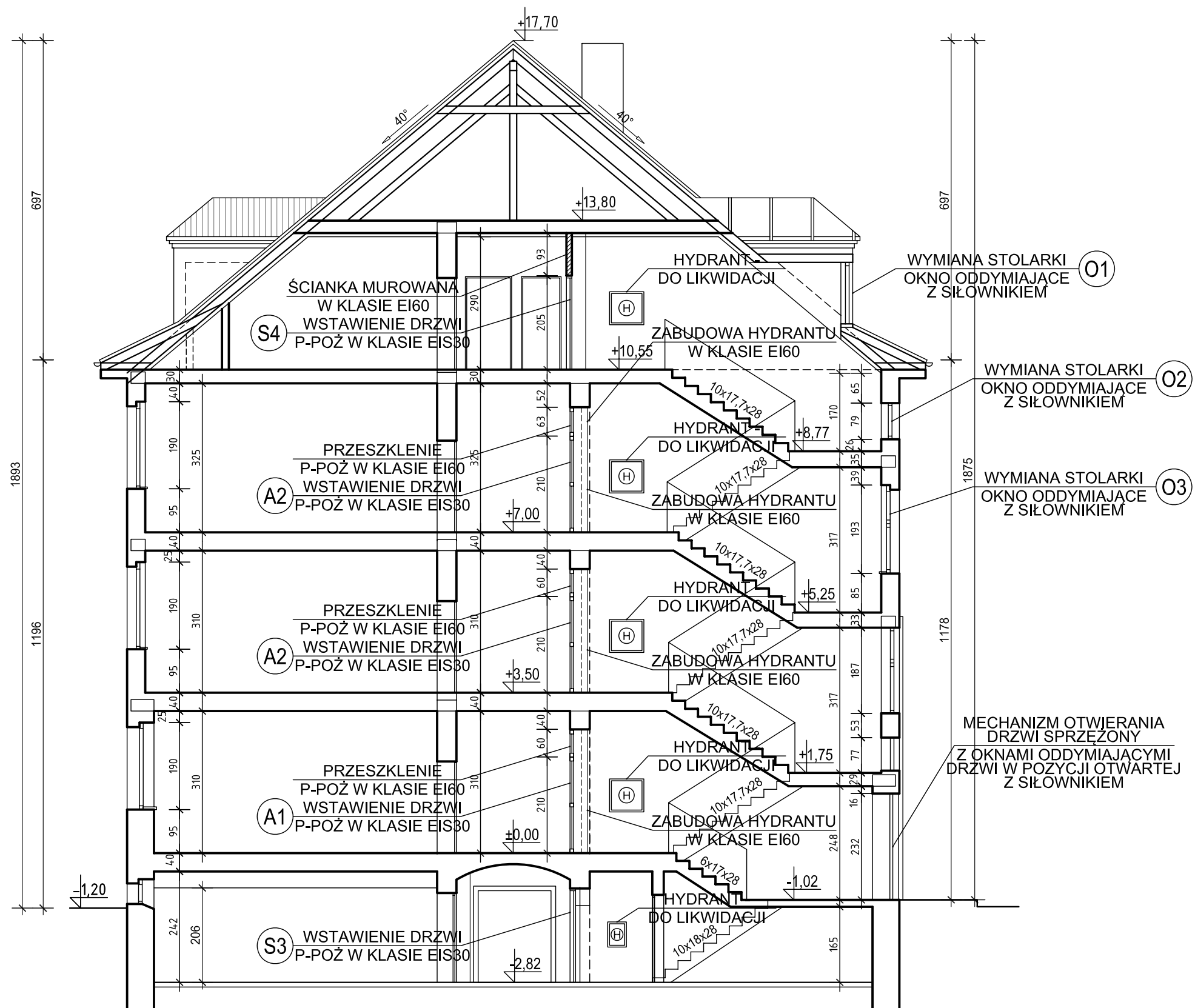
PRZEKRÓJ A - A - STAN PROJEKTOWANY 1:100 BUDYNEK "B"
