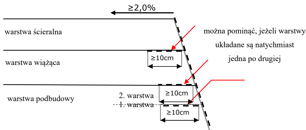
Rysunek 1. Wykończenie oraz uszczelnienie wyżej położonej krawędzi warstwy dla nawierzchni o jednostronnym nachyleniu
