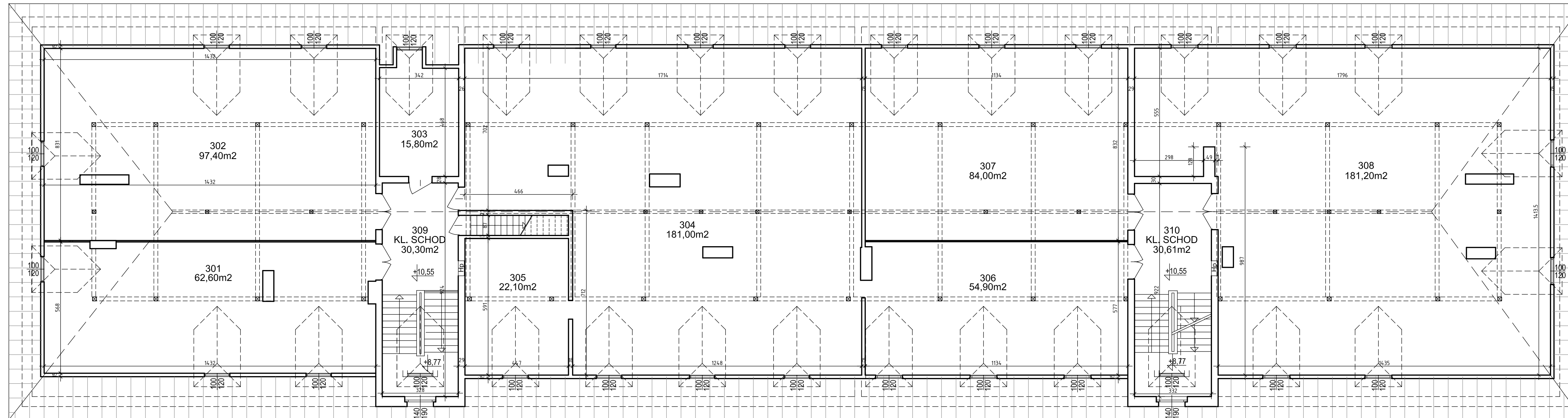
RZUT PODDASZA - STAN ISTNIEJĄCY 1:100 BUDYNEK "B"
