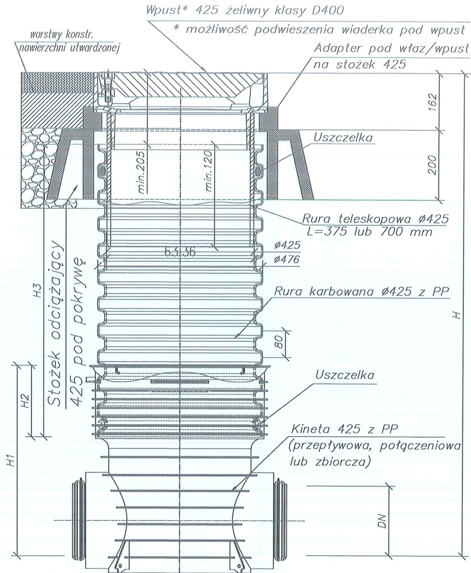
Studzienka inspekcyjna 425 z rurą teleskopową i wpustem klasy D400 na stożku odciążającym 425
