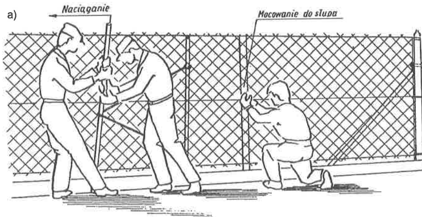
Rys. 9. Przykłady mocowania siatki do linek usztywniających (wg [6])
