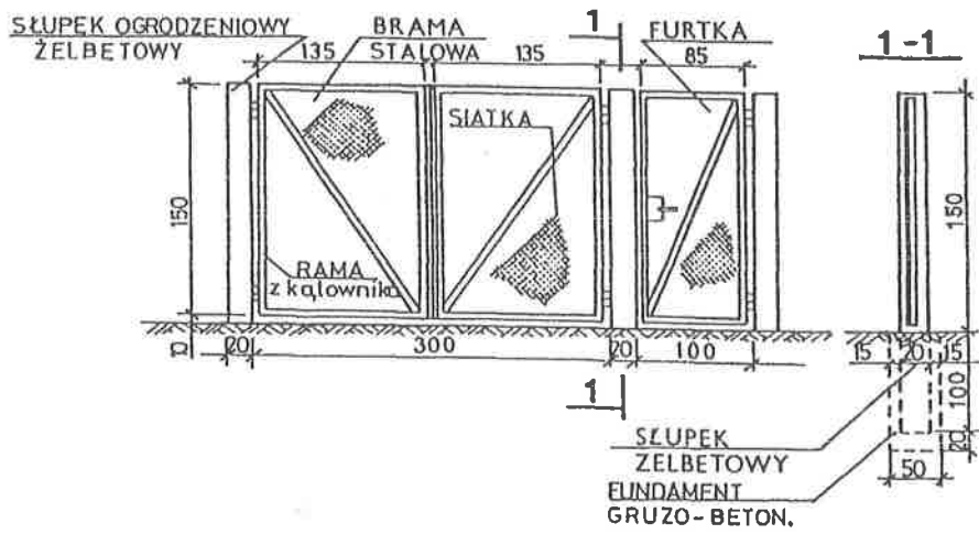
Rys. 10. Przykład bramy i furtki w ogrodzeniu (wg [5])
