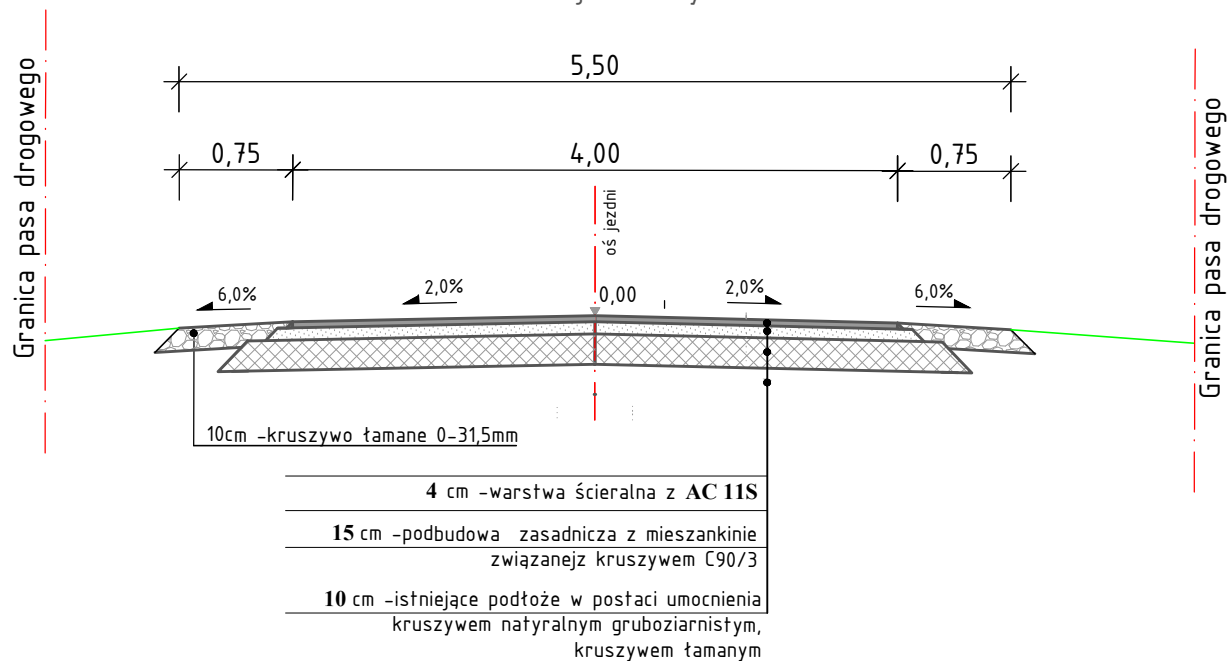
Przekrój normalny
