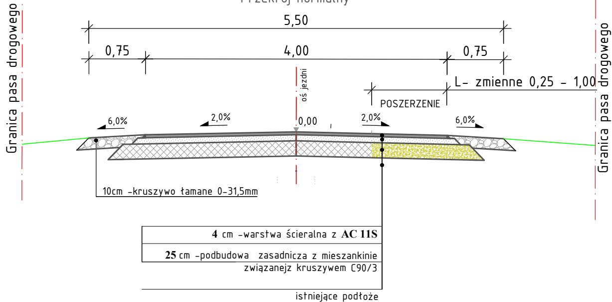
Przekrój normalny
