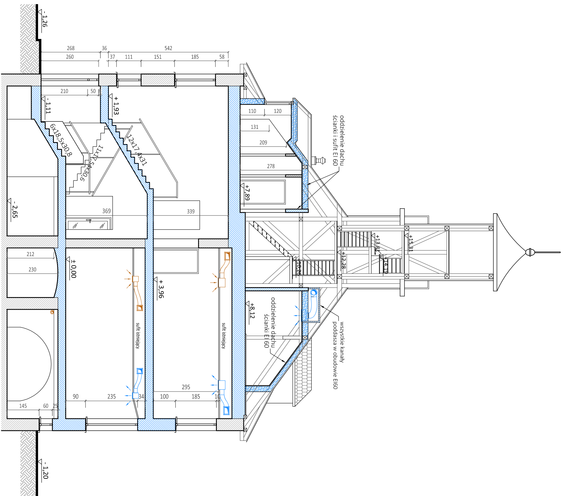
PRZEKRÓJ A-A skala 1:100
