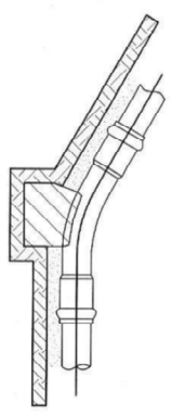
BLOK OPOROWY ŁUKU NA ZAŁAMANIU PRZEWODU W PIONE WARIANT I
