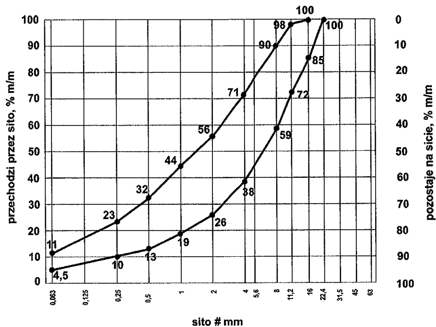
Rys. 1 Uziarnienie mieszanki CBGM 0/16mm
