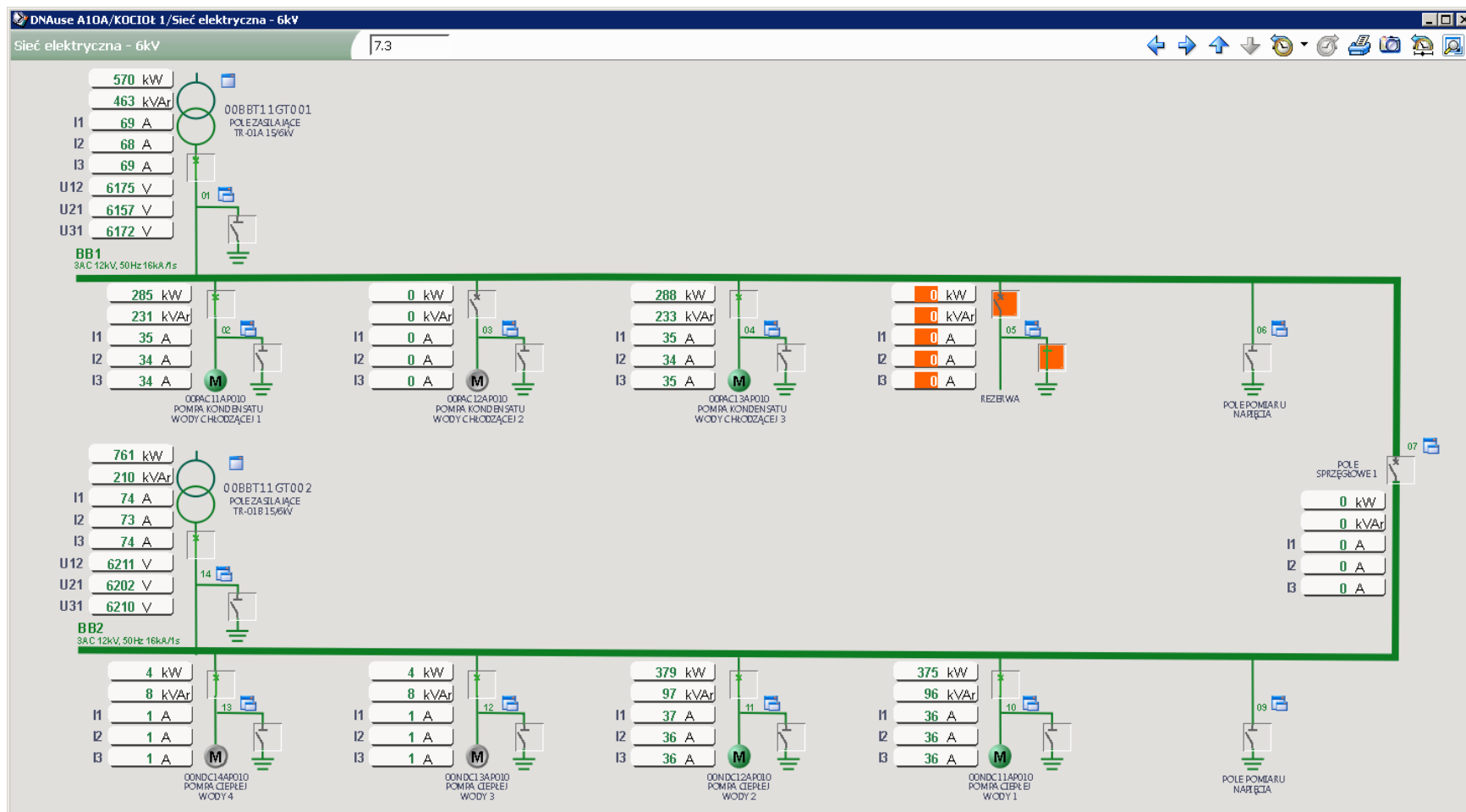
Rysunek 3.21 Zrzut ekranu systemu kontroli eksploatacji przedstawiający schemat sieci elektrycznej 6kV w ZTPO
