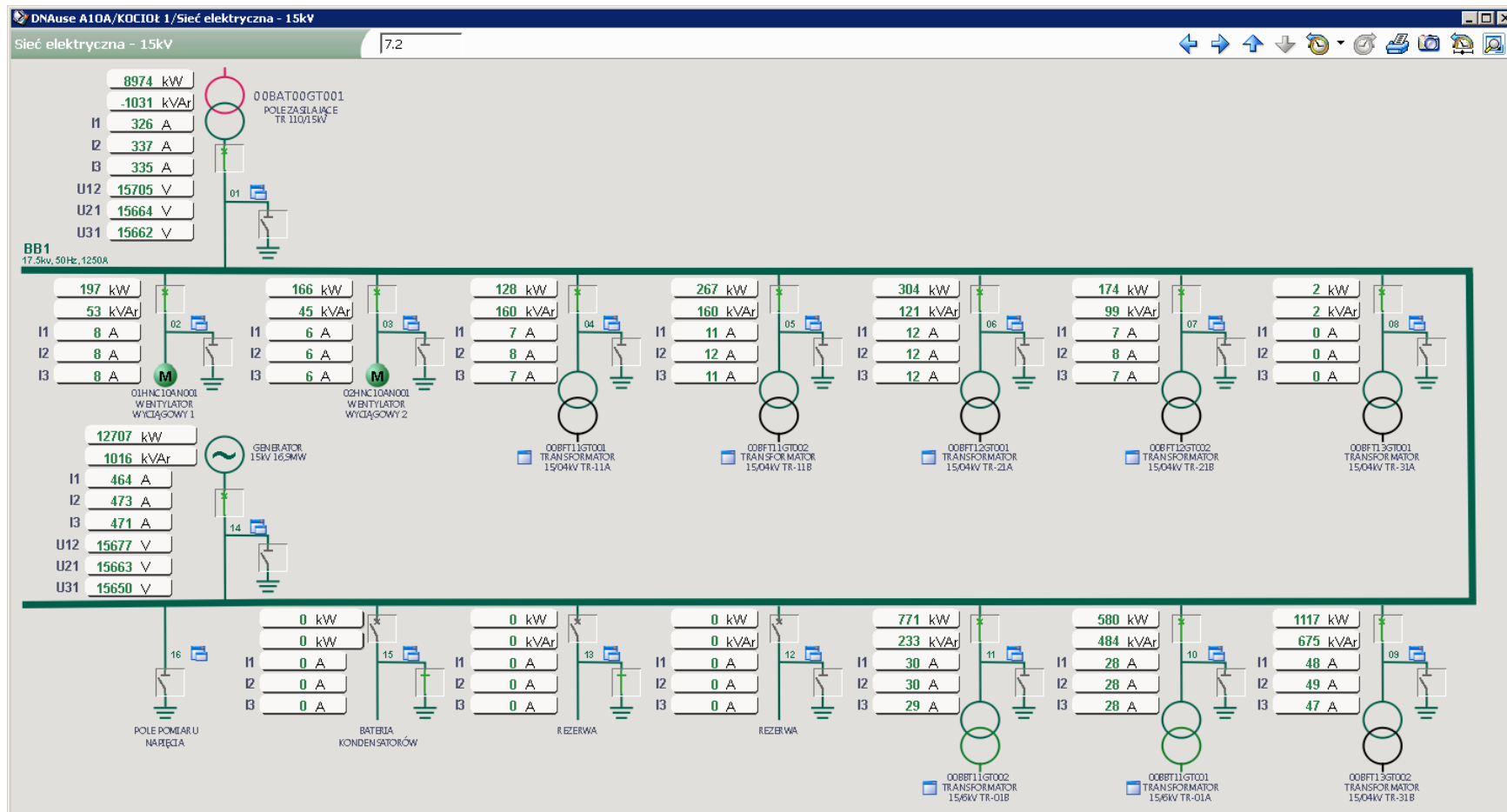
Rysunek 3.20 Zrzut ekranu systemu kontroli eksploatacji przedstawiający schemat sieci elektrycznej 15kV w ZTPO
