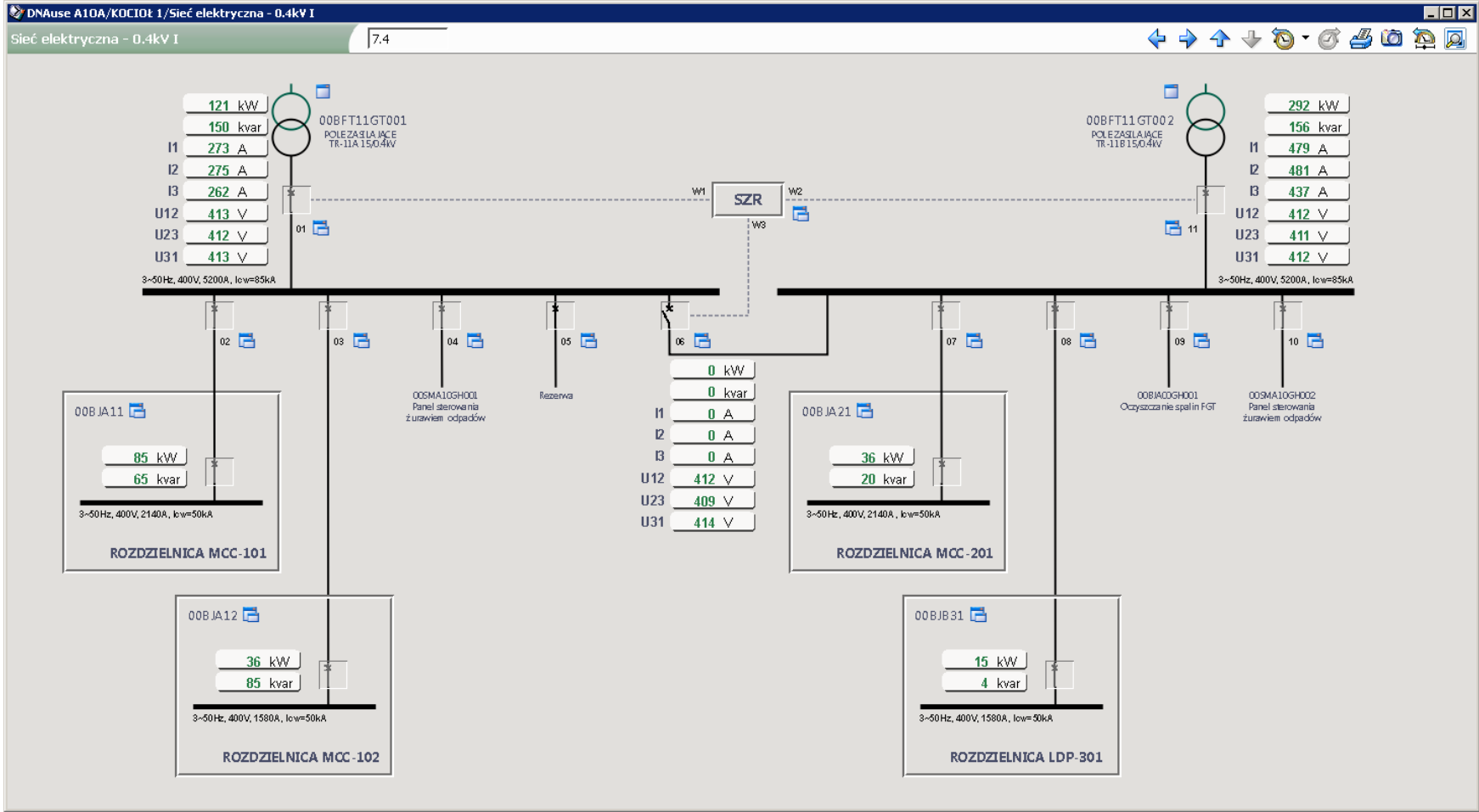
Rysunek 3.22 Zrzut ekranu systemu kontroli eksploatacji przedstawiający schemat rozdzielni I 0,4kV w ZTPO
