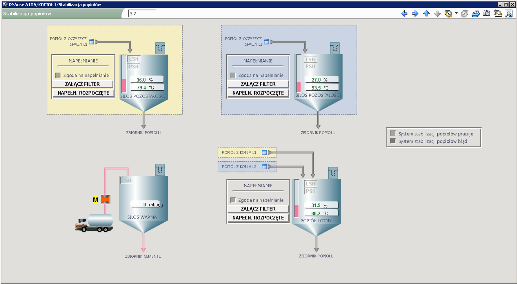
Rysunek 3.18 Zrzut ekranu systemu kontroli eksploatacji przedstawiający system stabilizacji popiołów
