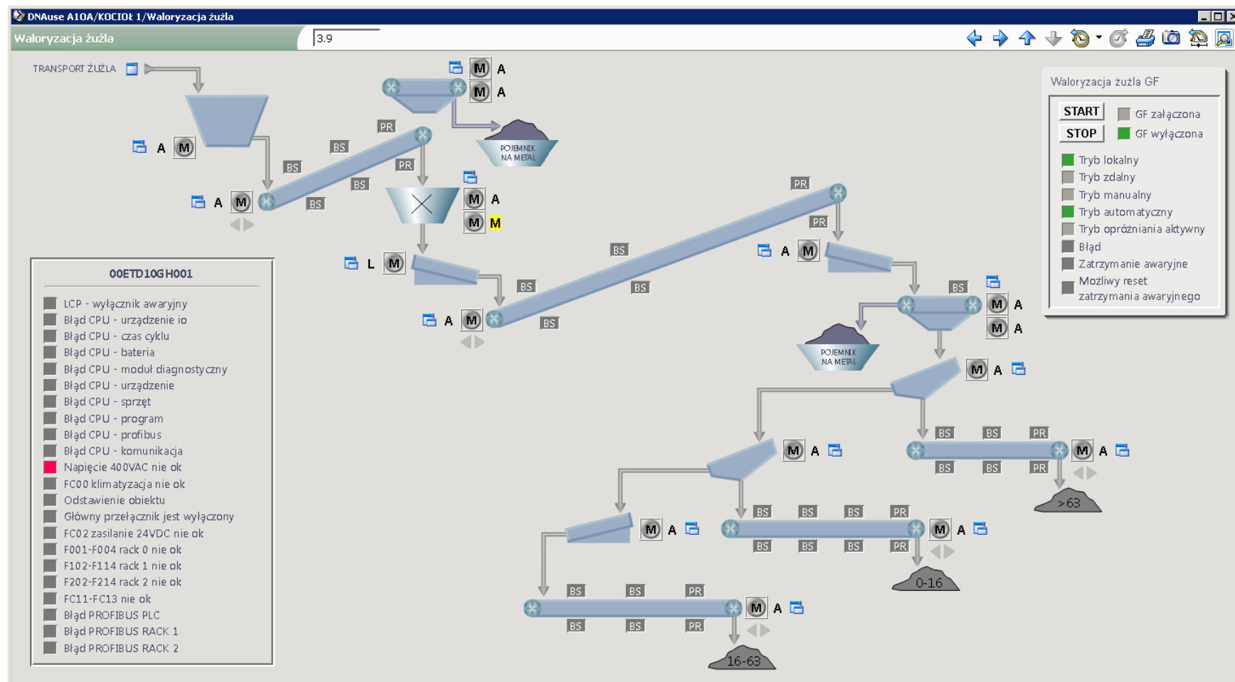
Rysunek 3.17 Zrzut ekranu systemu kontroli eksploatacji przedstawiający Węzeł Waloryzacji Żużla
