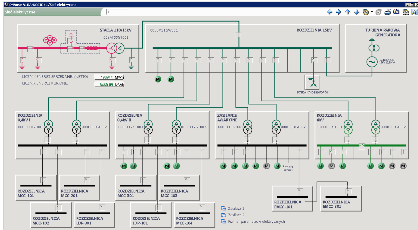
Rysunek 3.19 Zrzut ekranu systemu kontroli eksploatacji przedstawiający sieci elektrycznej w ZTPO
