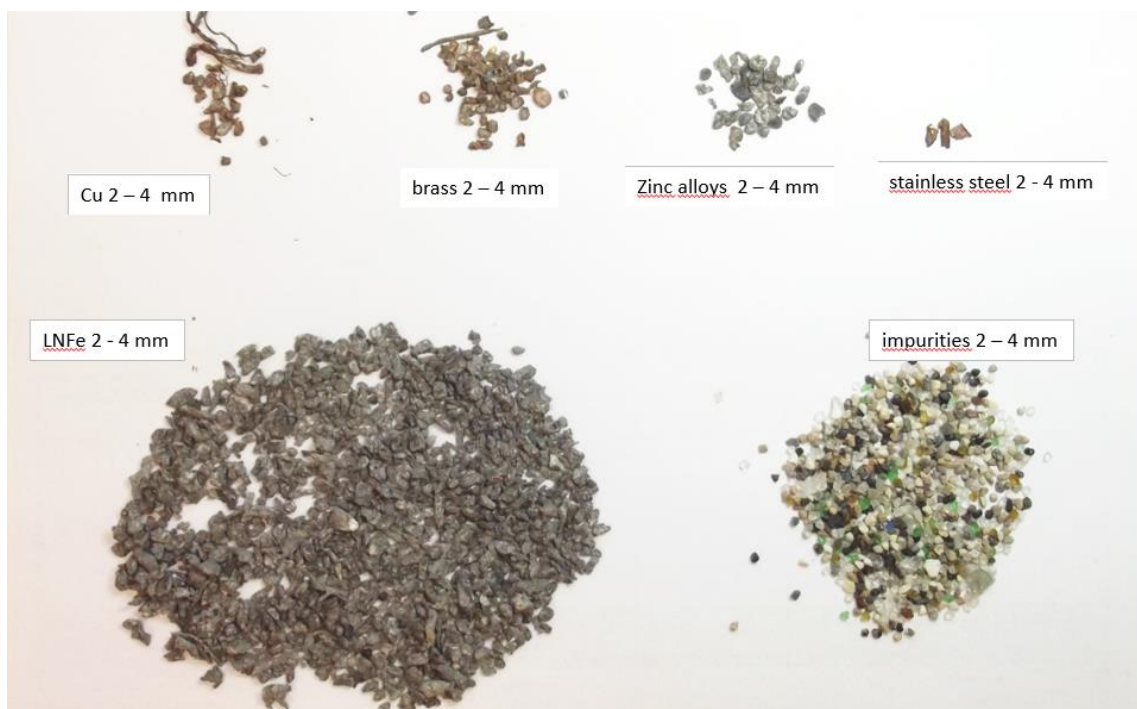
Rysunek 3.7 Przykłady form występowania metali i zanieczyszczeń o frakcji 2 – 4 mm.
