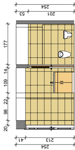
WIDOK J3
