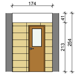
WIDOK M3
